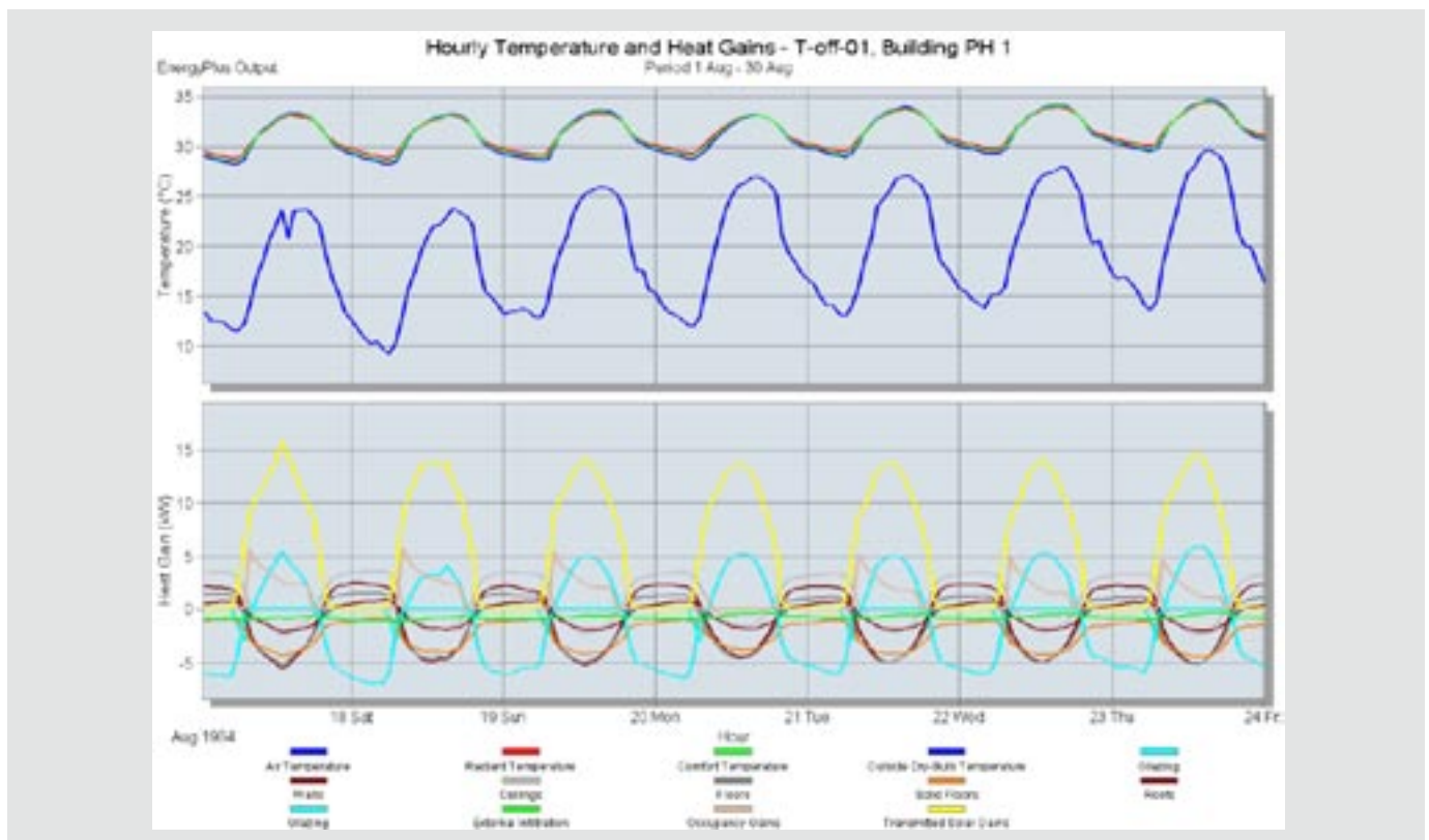
Bild 40: Grafische Ausgabe von Simulationsergebnissen für eine Sommerwoche, hier ein Beispiel mit unzureichendem Sonnenschutz, gerechnet mit meteorologischen Testdaten aus dem Jahr 1984
