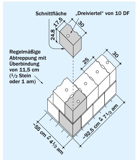
Bild 12 Ecke von 30 cm dicken Wänden aus 10 DF (300)-Steinen mit ½- und ¾-Steinen zum Ausgleich
