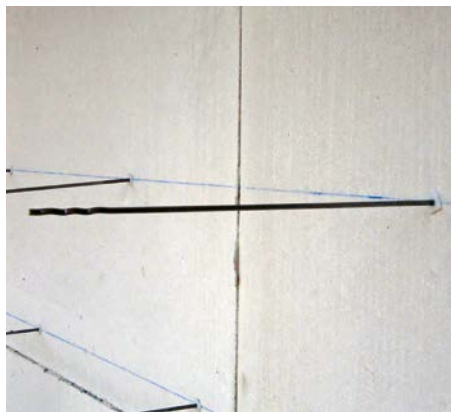
Bild 14 In die Tragschale eingedübelte Luftschantanker
