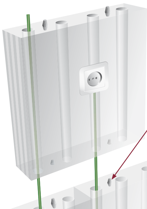
Detail: Zentrierbolzen
