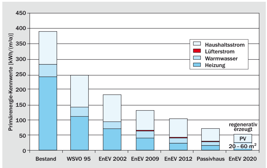
Primärenergie-Kennwerte von Baustandards
