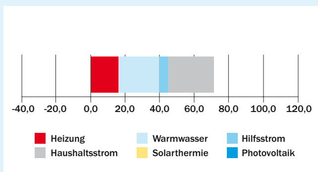
Primärenergiebilanz (Bereiche Heizung, Warmwasser und Hilfsstrom weisen eine Plusenergiebilanz auf)
