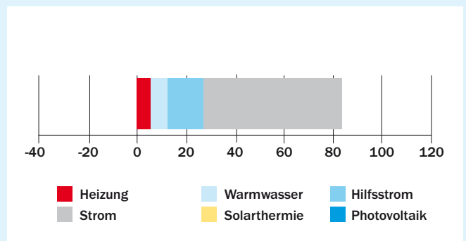
Primärenergiebilanz
