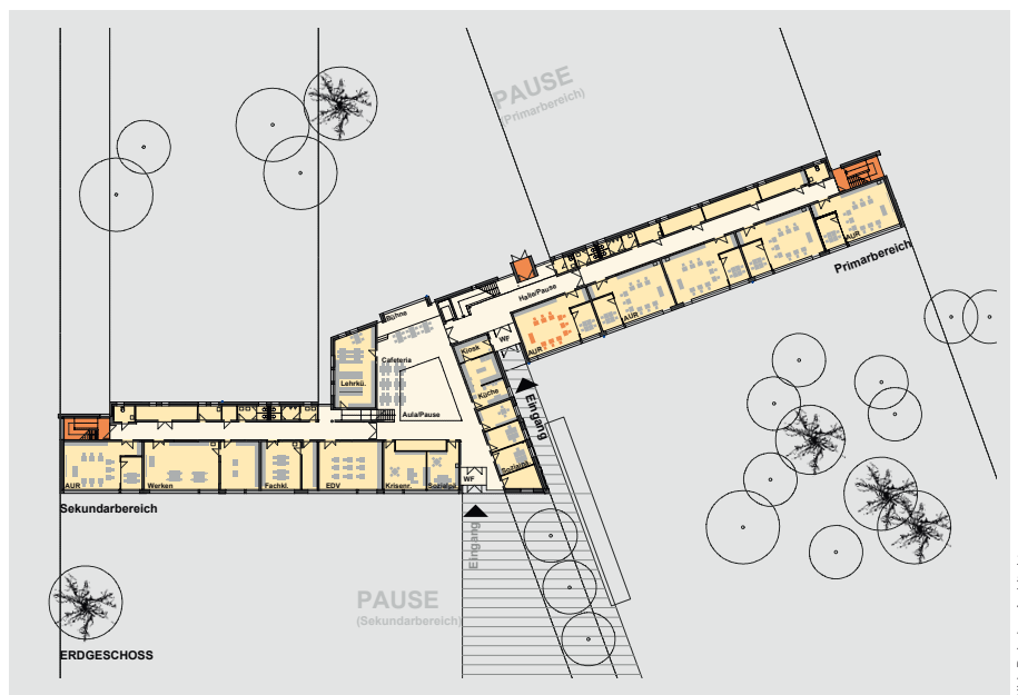
Grundriss EG
