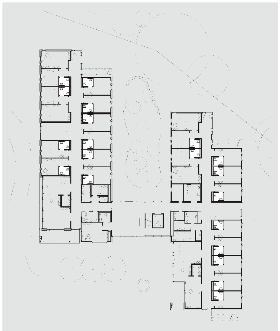
Grundriss EG
