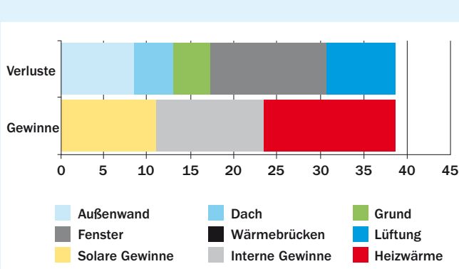
Energetische Bilanzierung des Heizwärmebedarfs: Gewinne und Verluste [kWh/(m²a)]
