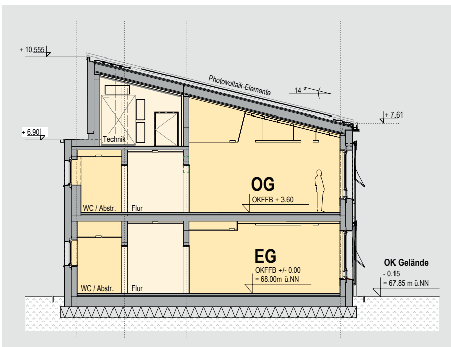
Schnitt
