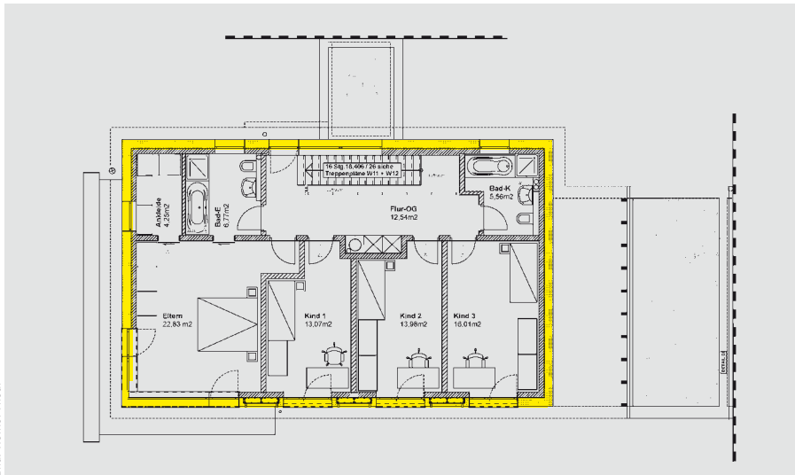
Grundriss OG
